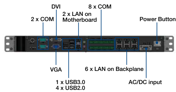
后视图#2
