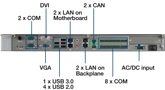
后视图#1
