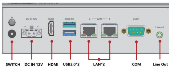
前视图
