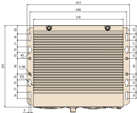
RIRR-IPC-BOX-H420-A2-210 机身长度210mm
